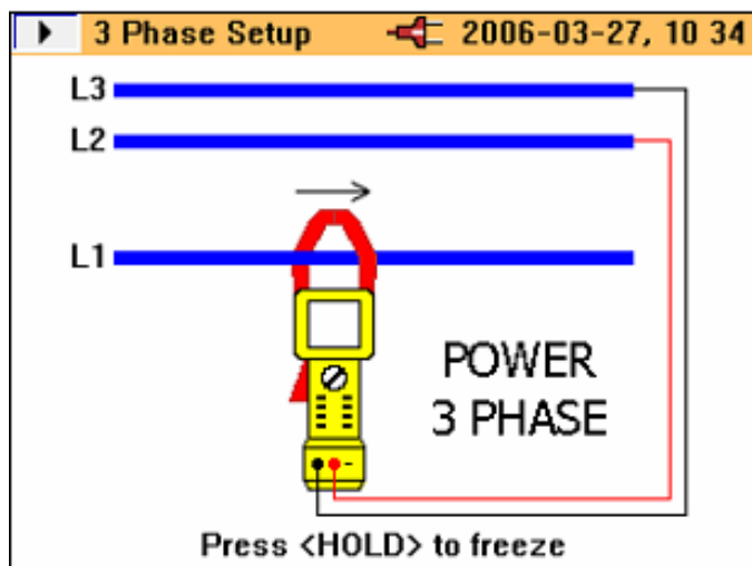
图 9. 三相电力网的测量连接
