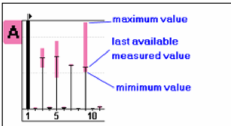
图 16. 谐波记录画面的详细视图
