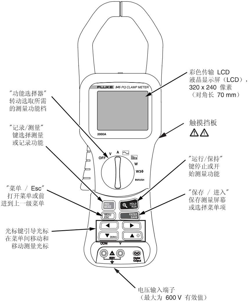
图 4. 345 正视图
