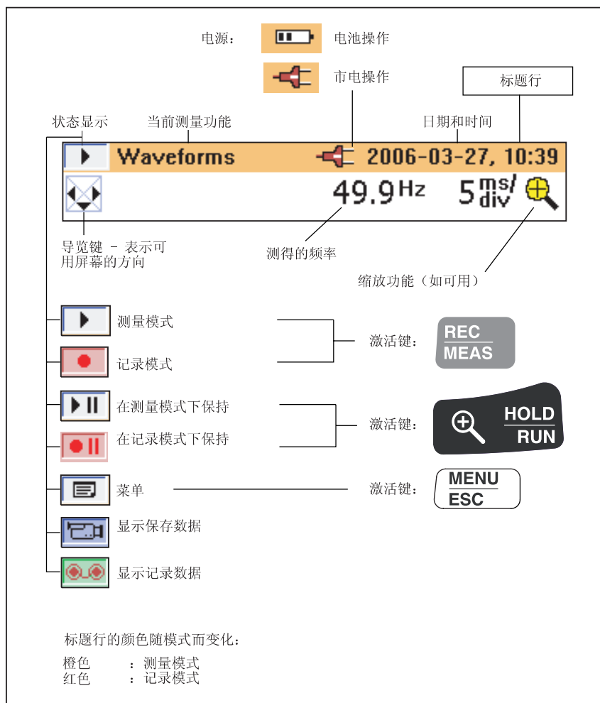
图 10. 钳表的显示符号
