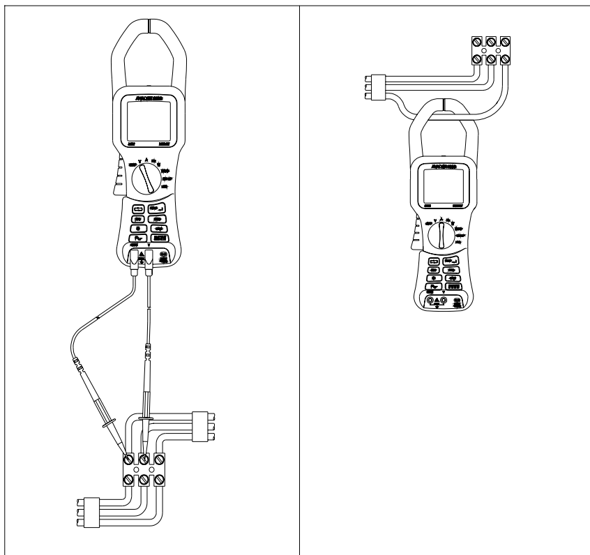
图 7. 电压和电流测量连接
