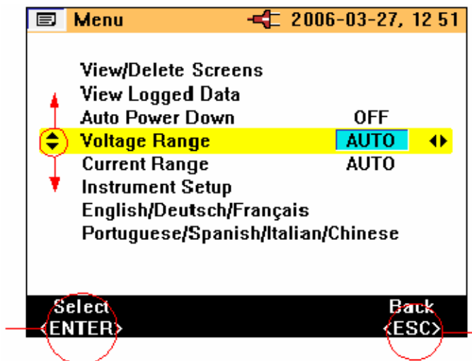
图 11. 显示屏导览
