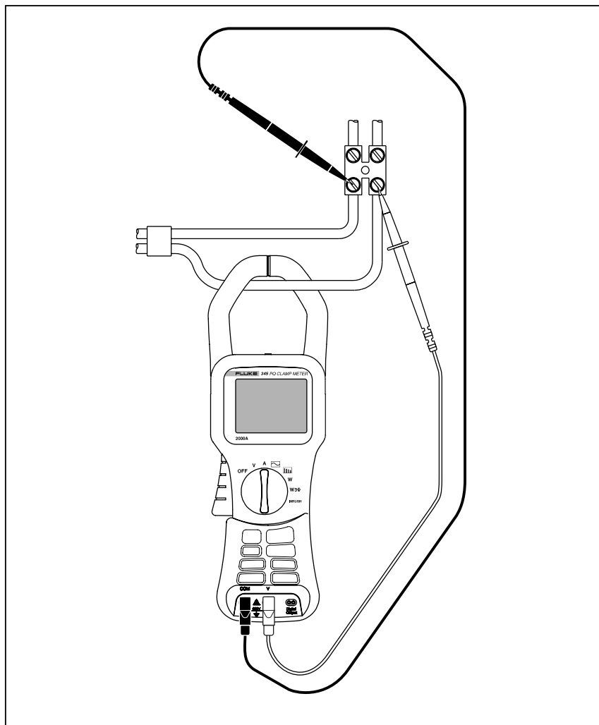
图 8. 单相电力网的测量连接
