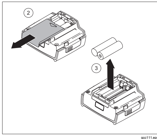
图 10. 取下显示模块电池
