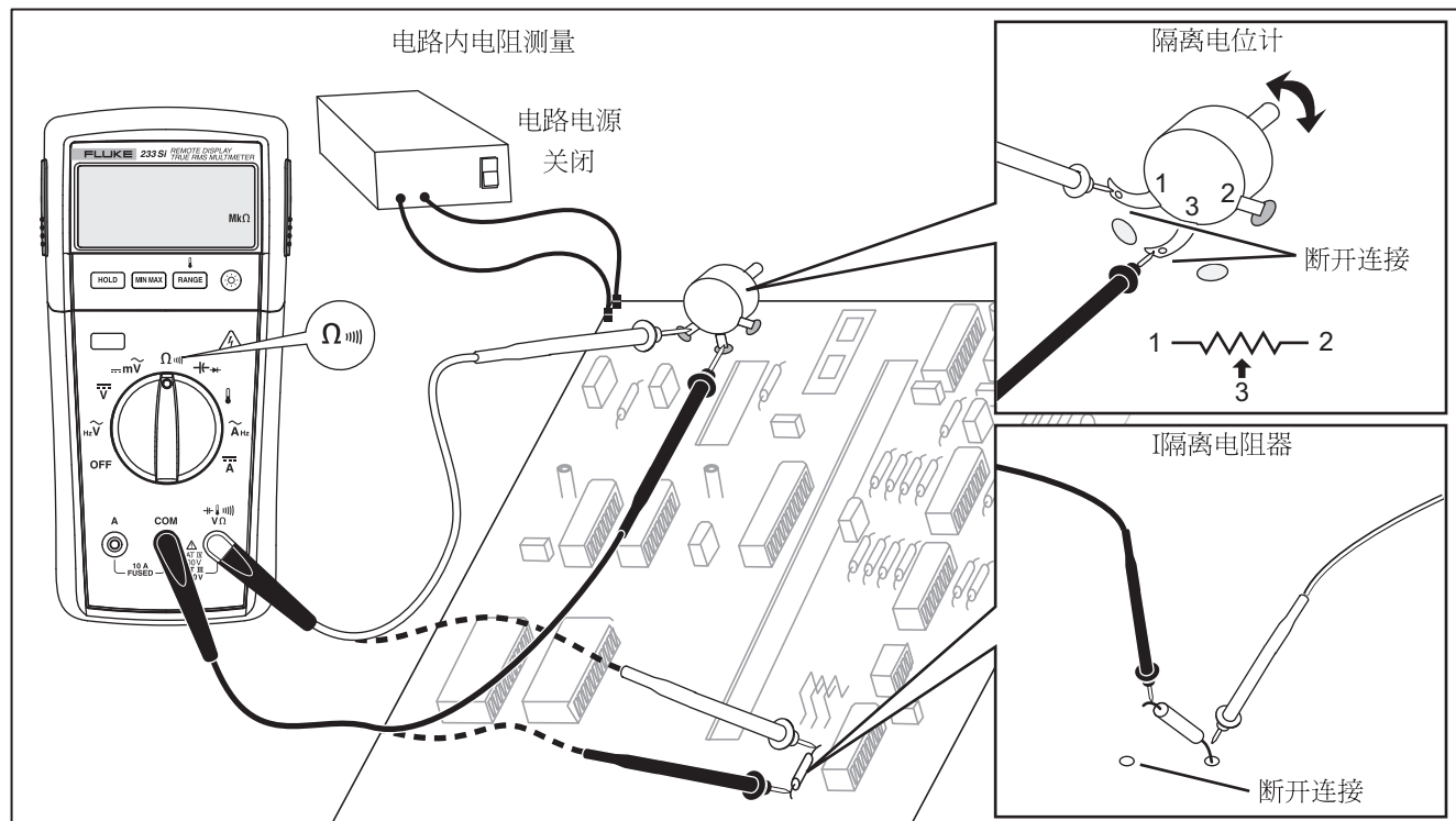
图 2. 电阻测量
