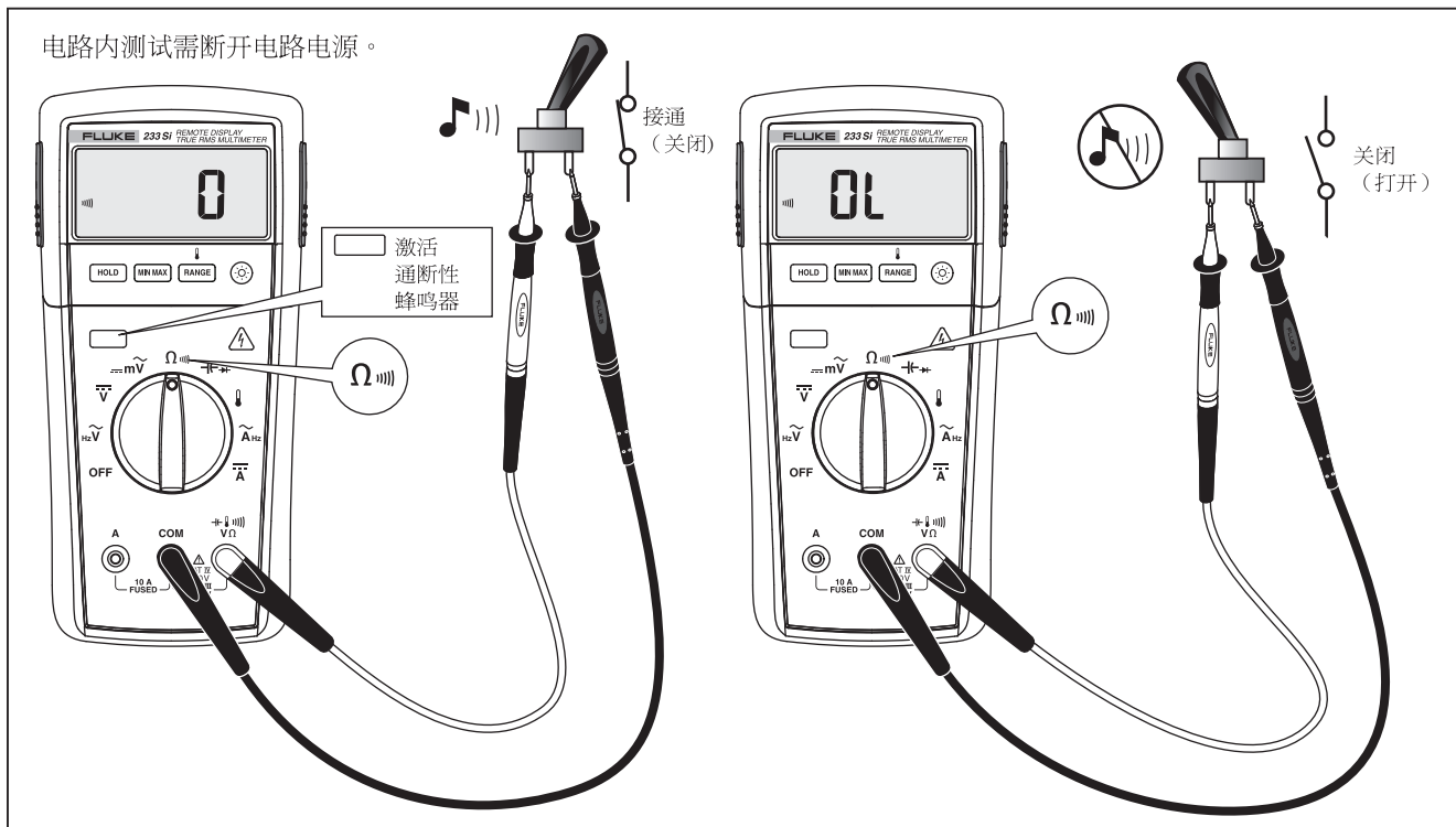
图 3. 通断性测试
