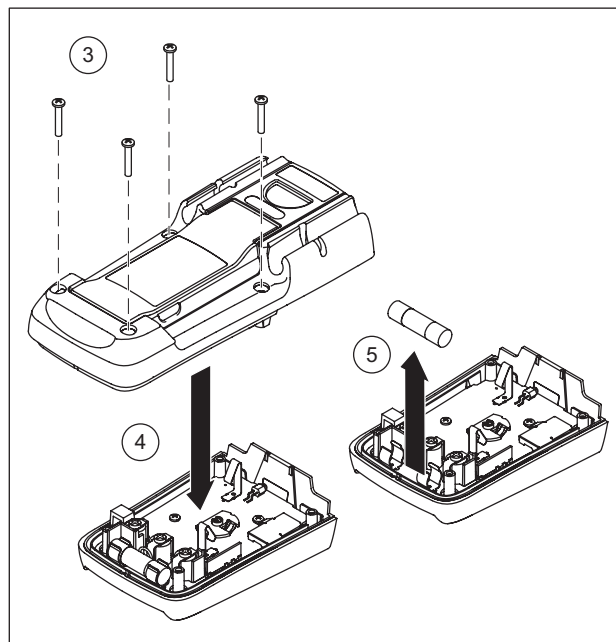
图 12. 更换保险丝
